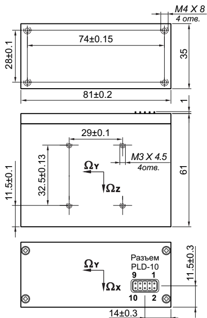
ГАБАРИТНО - УСТАНОВОЧНЫЙ ЧЕРТЕЖ
