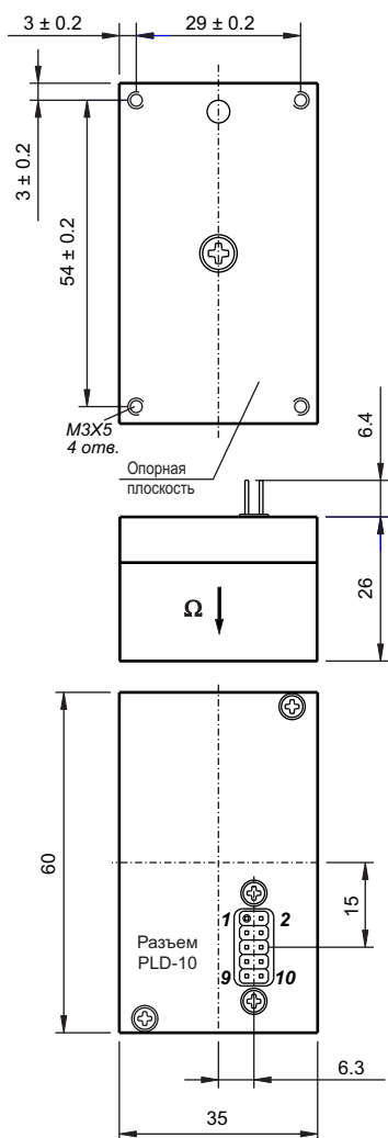
ГАБАРИТНО - УСТАНОВОЧНЫЙ ЧЕРТЕЖ
