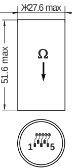
ВГ091Б-300, ВГ091Б-200Ш
