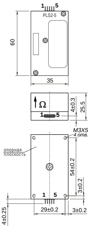
ВГ095Д
