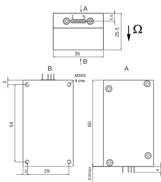
ВГ941-3АМ-02
