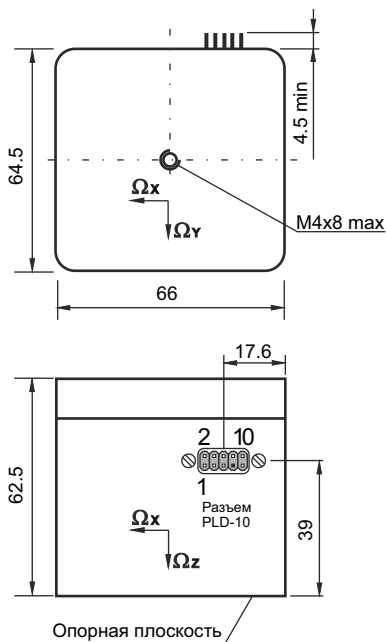
ГАБАРИТНО - УСТАНОВОЧНЫЙ ЧЕРТЕЖ
