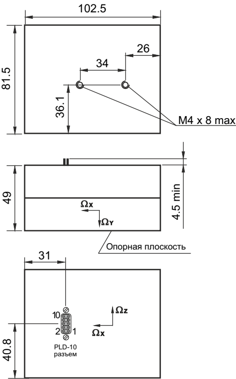
ГАБАРИТНО - УСТАНОВОЧНЫЙ ЧЕРТЕЖ
